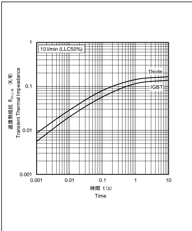
過渡熱抵抗特性 Transient Thermal Impedance Characteristics
